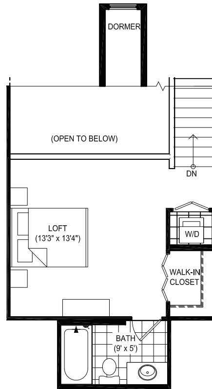
LOFT
